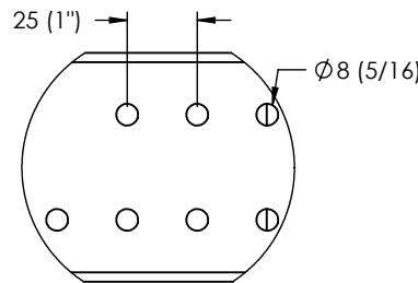
DETALLE E DISTANCIA DE PROFUNDIDAD VARIABLE
