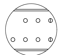
DETALLE A Perforaciones para ajuste de profundidad.
